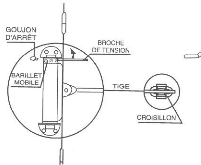
PORTE A DROITE barillet mobile placé en haut
