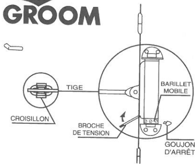
PORTE A GAUCHE barillet mobile placé en bas
